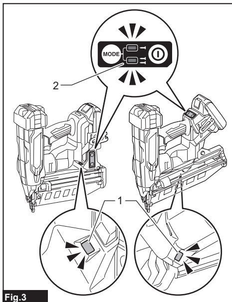
Fig.3 ► 1. Lampe 2. Indicateur d'alimentation/mode
